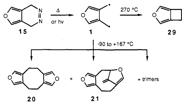
Scheme VI
